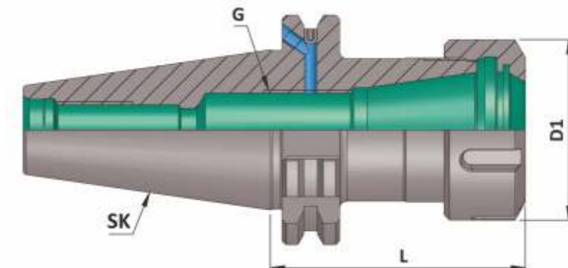
SK (DIN 69871) Collet Chuck ER (AD+B) AD/AF
