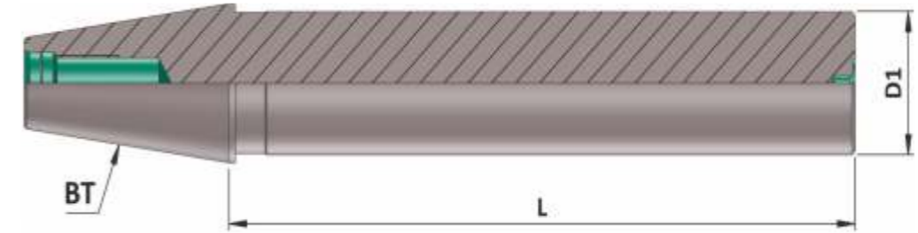
BT (MAS 403) Master Mandrell
